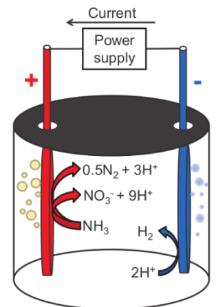
Figure 8 : Traitement basique par électro-oxydation (oxydation de l'azote ammoniacal) Source : VUNA, EAWAG
