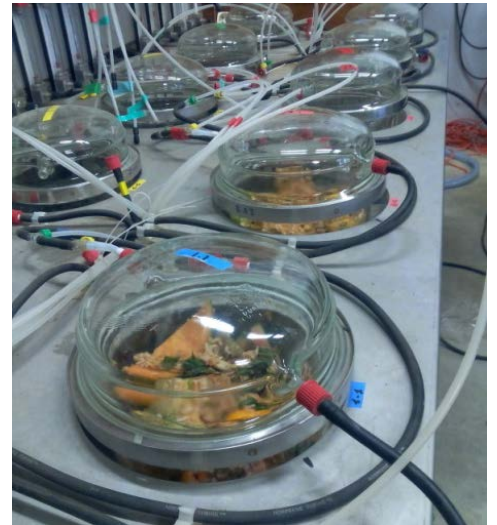
Figure 5 : Dégradation de la matière organique : suivi des dégagements gazeux
